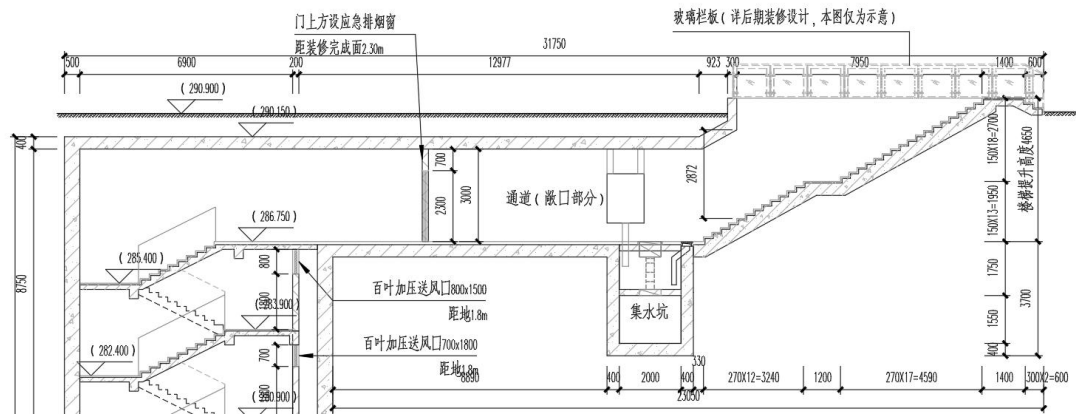
安全出口剖面图
